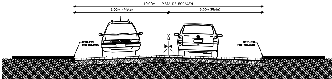
SEÇÃO TIPO DE BLOCO INTERTRAVADO - RUA GUIDO WAECHTER
